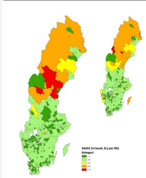
Figur 24 Genomsnittlig avbrottsid per kund (SAIDI) per redovisningsenhet 2021 (miniatyrkarta för jämförelse med 2020)
